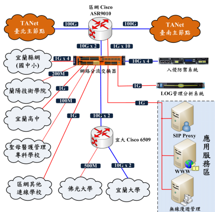
圖 19. 宜蘭區網中心架構示意圖
