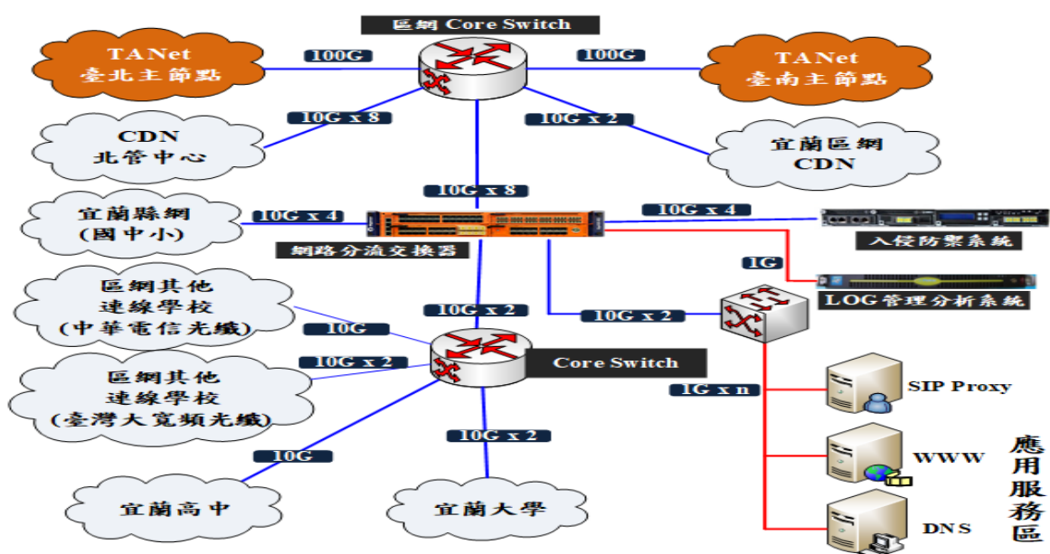
圖 19. 宜蘭區網中心架構示意圖
